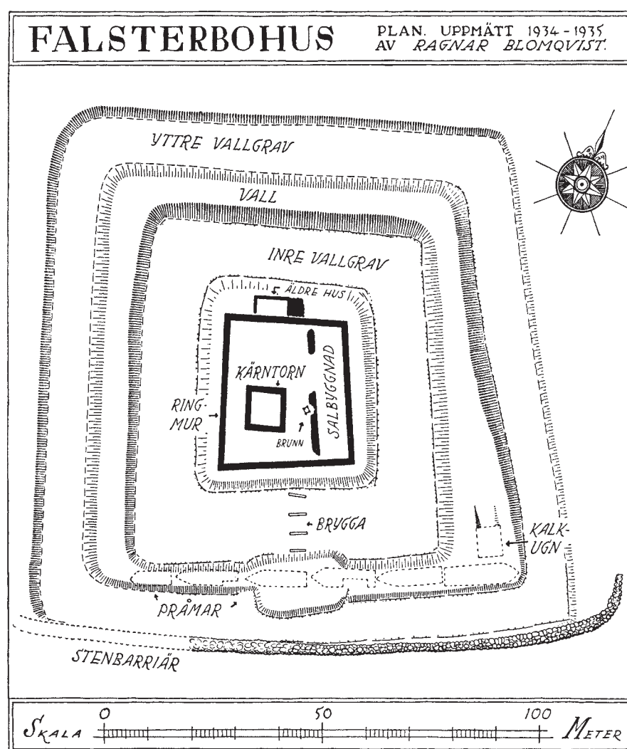
Planritning Falsterbohus. Efter Blomqvist, R: "Falsterbohus". Kulturens årsbok, Lund 1950.
